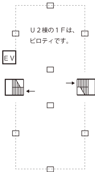
1 F 平面図
